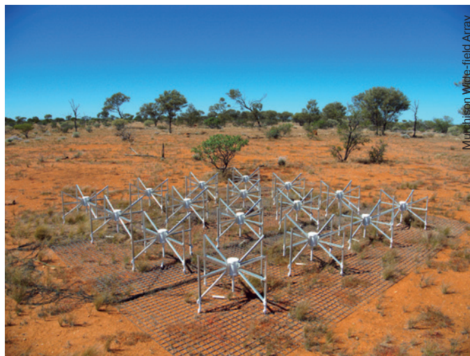
▲ Одна из «плиток» радиотелескопа Мерчинсона (MWA), построенного в Австралии. В рамках подготовки к поиску галактик первого поколения опубликован первый каталог внегалактических источников излучения метрового диапазона, полученный с помощью уже работающих элементов телескопа.
