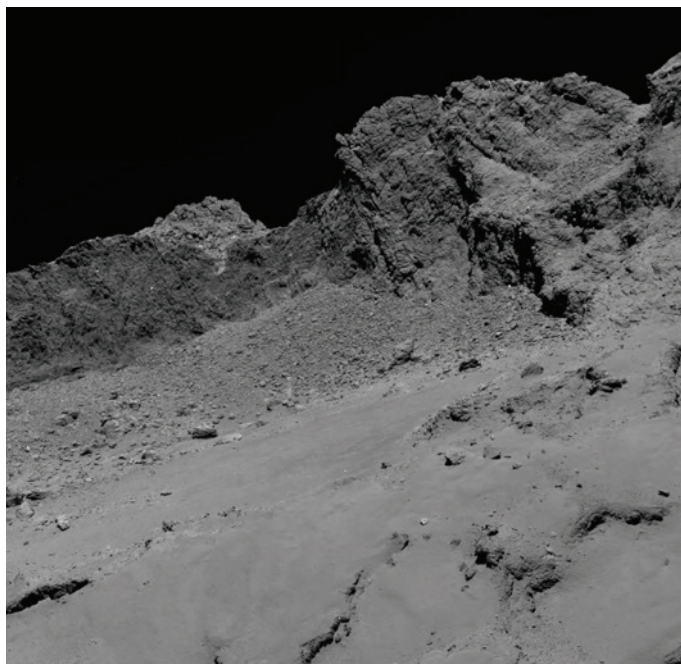
▲ Фотография кометы Чурюмова-Герасименко, сделанная камерой OSIRIS европейского аппарата Rosetta 30 сентября 2016 г. в 01:20 UTC с высоты около 16 км. Сторона снимка имеет размер около 615 м, разрешение достигает 30 см на пиксель.
