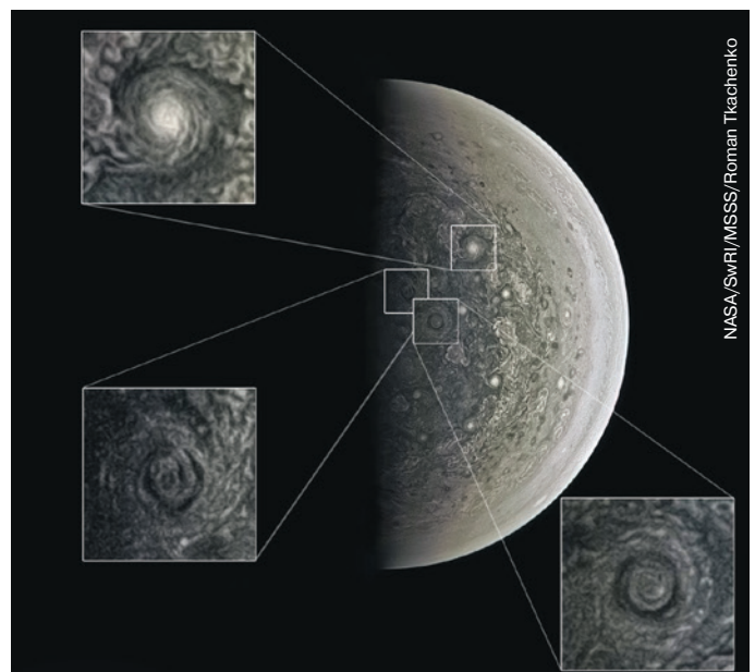
▲ Вихревые облачные структуры, сфотографированные зондом Juno в окрестностях южного полюса Юпитера при последнем прохождении перигея — в конце августа 2016 г. По размерам эти структуры сравнимы с нашей Луной.
